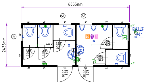
Prefabbricato modulare ad uso WC, donne/uomini, da 20'
