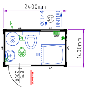
Prefabbricato modulare ad uso WC e doccia da 8'
