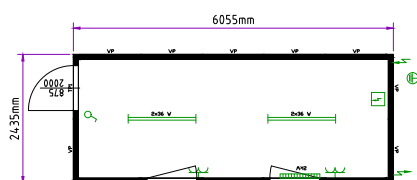
Prefabbricato modulare ad uso ufficio da 20' standard
