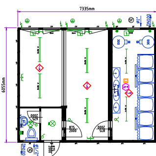
Prefabbricato modulare ad uso ufficio e sanitario, impianto da 3 unità
