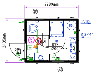
Prefabbricato modulare ad uso sanitario da 10'
