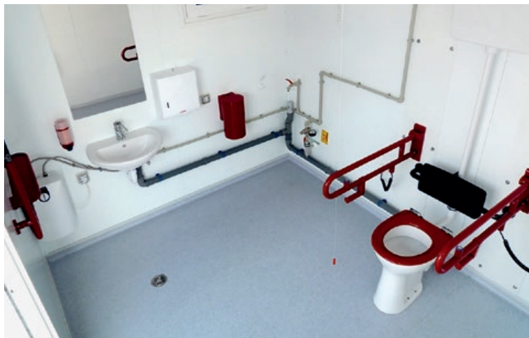
Vista interna modello per disabili secondo DIN 18040-1
