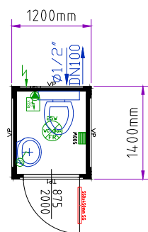
Prefabbricato modulare ad uso WC da 5'
