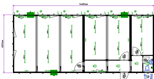
Prefabbricato modulare ad uso ufficio e sanitario, impianto da 6 unità
